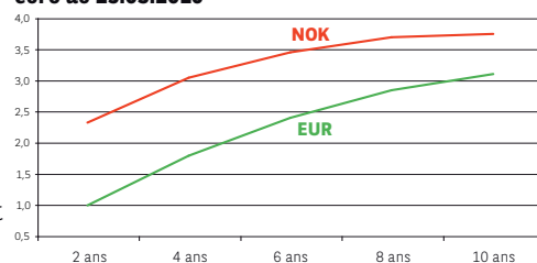
Courbe des taux norvégiens et de ceux de la zone euro au 25.03.2010
