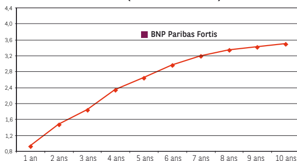
Courbe des taux en euro (Bunds allemands 1 ) au 22/06/2009
